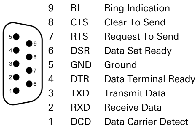
Abbildung 5: RS232-Schnittstelle
